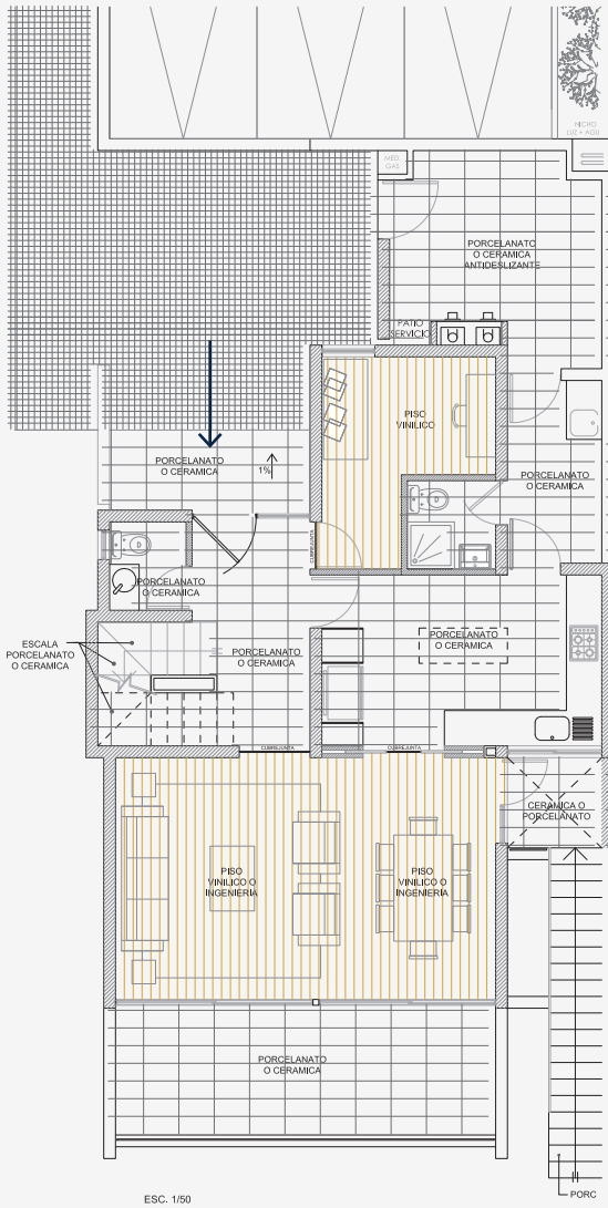
PLANTA PRIMER PISO Casa tipo
